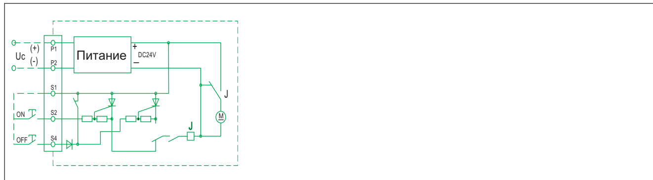
схема подключения моторного привода(AC)
